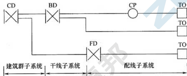
图 3.1.2-2 综合布线子系统构成
